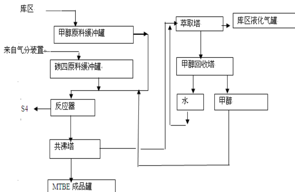
图 2.2—3 (4) MTBE 装置工艺流程及产污环节图
