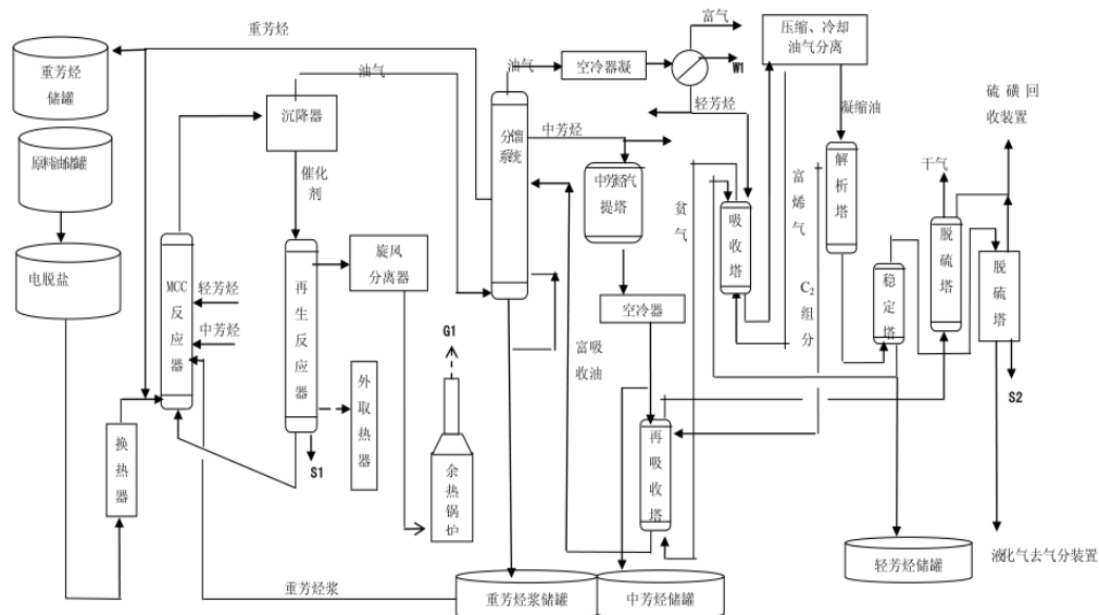
图 2.2-2 (1) MCC 装置工艺流程示意图
